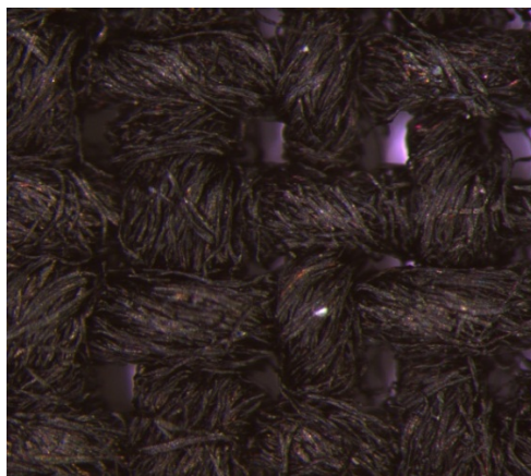
Рисунок 7 — Бязь, нагретая при температуре 400 °С при увеличении 10 х (А) и 50 х (Б)
