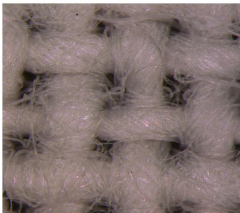
Рисунок 3 — Бязь, нагретая при температуре 200 °С при увеличении 10 х (А) и 50 х (Б)
